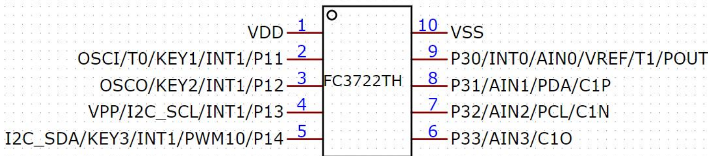
10PIN 管脚分布
