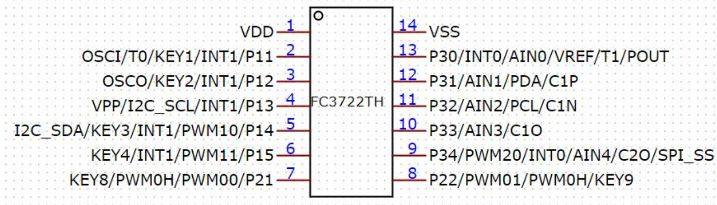
14PIN 管脚分布
