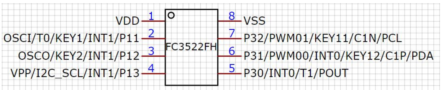
图 3 8PIN 管脚图
