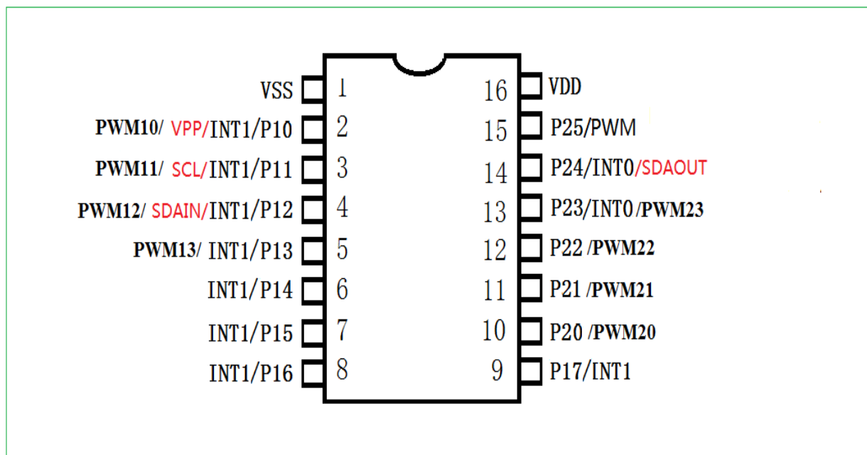
图 1 16 PINS 管脚分配
